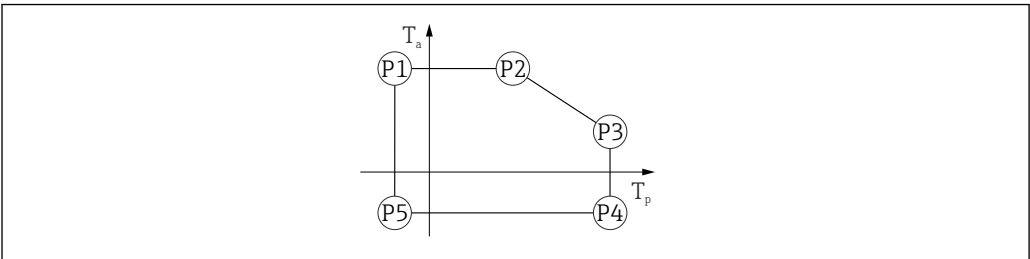
29 316L 外壳材质；过程温度范围：-40 ... +150 °C (-40 ... +302 °F)
