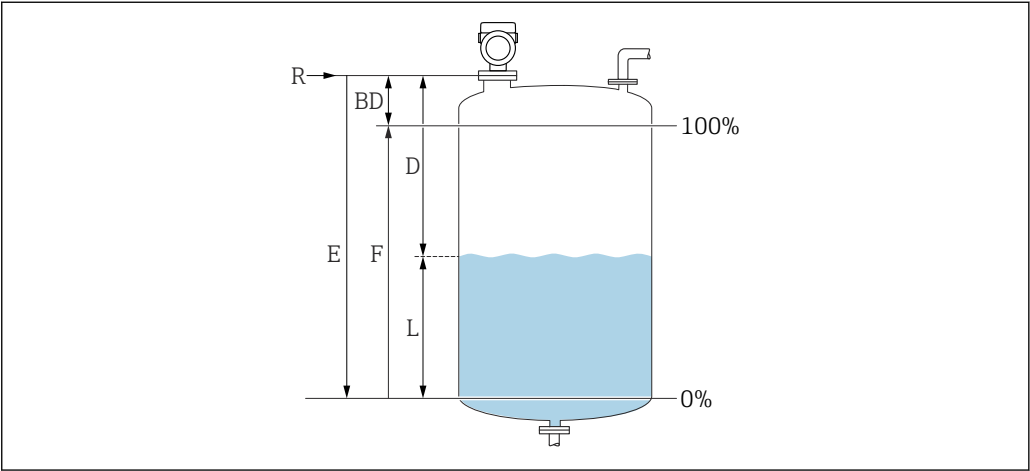
图 10 液位测量的设置参数
