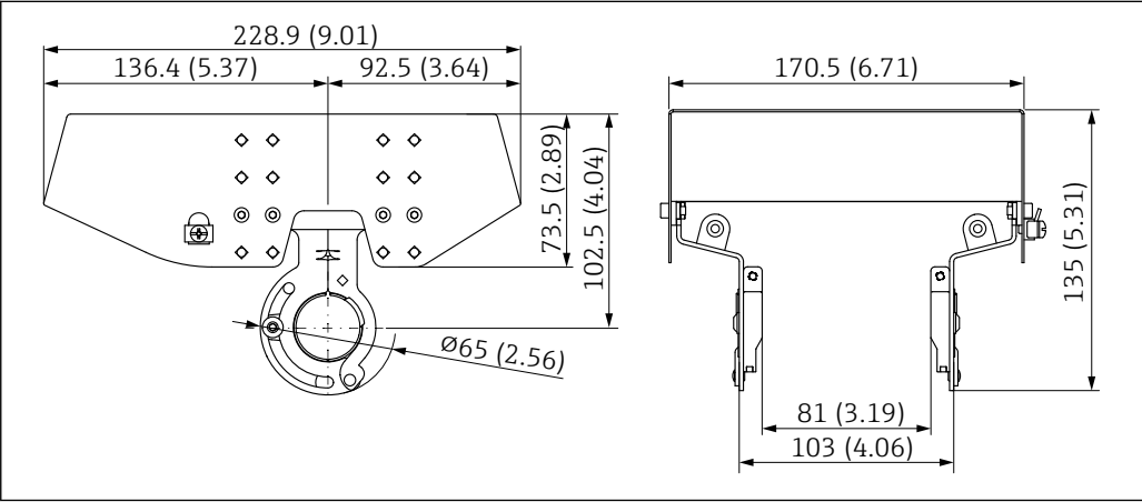
图 13 外形尺寸示意图。测量单位 mm (in)
