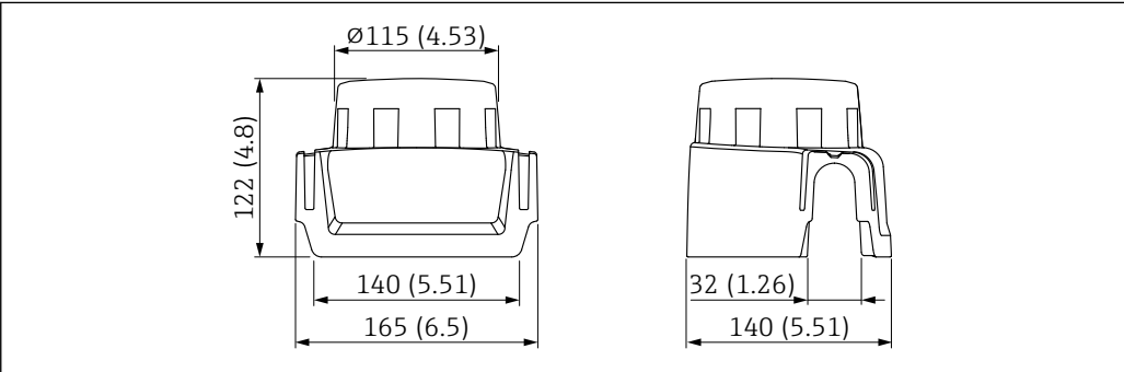
图 14 外形尺寸示意图。测量单位 mm (in)
