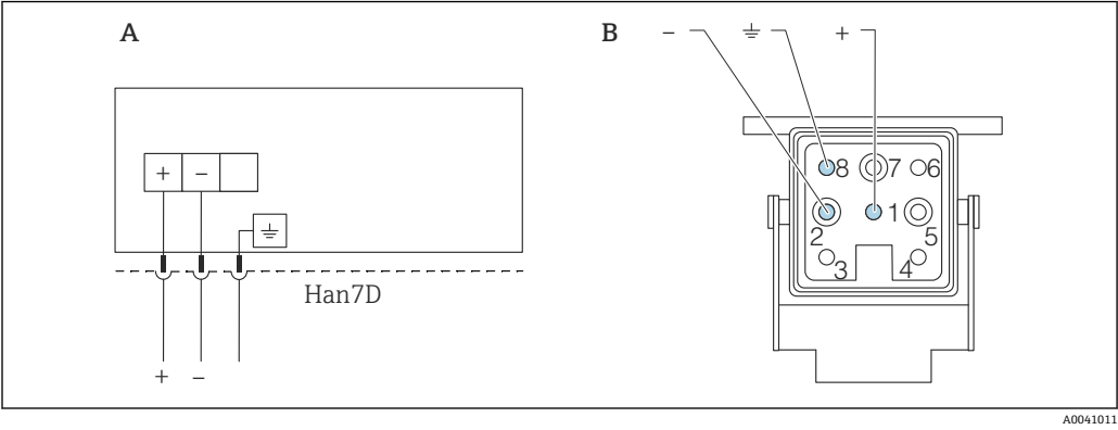
A 带 Harting Han7D 插头的仪表的电气连接示意图 B 仪表连接插头视图 - 棕色 ⏏ 黄/绿相间 + 蓝色
