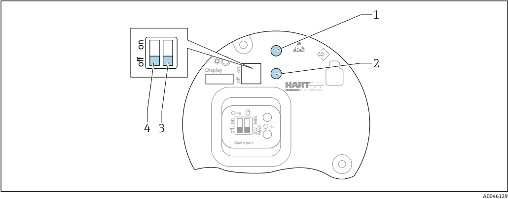
图 7 HART 电子插件上的操作按键和 DIP 开关
